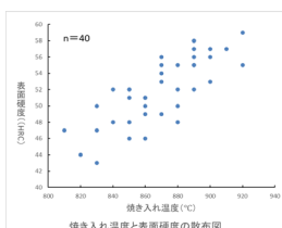
散布図
